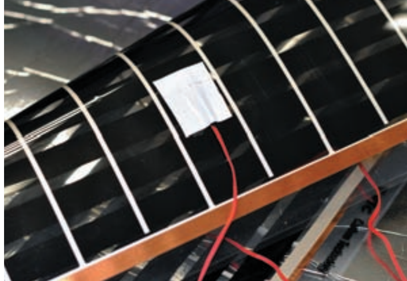
Рис. 25. Установленный и приклеенный датчик температуры пола. Вид снизу термопленки
