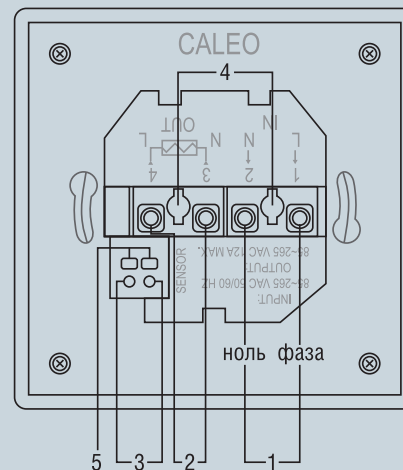
Рис. 21. Пример подключения соединительных проводов к терморегулятору CALEO UTH-10E
